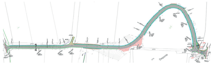
Darstellung Trassenverlauf
